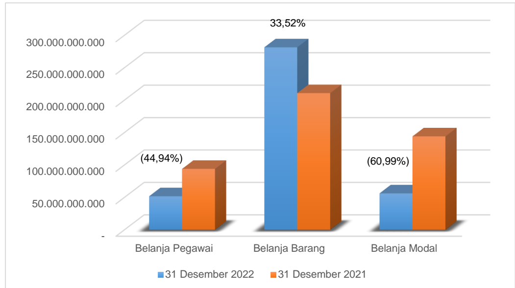
Gambar 5 Perbandingan Realisasi Belanja s.d. 31 Desember 2022 dan 31 Desember 2021
